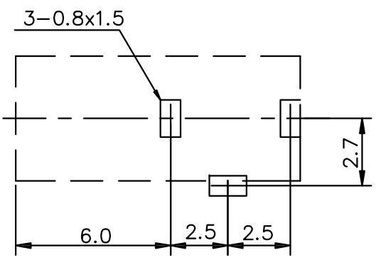
线路板安装尺寸示意图
