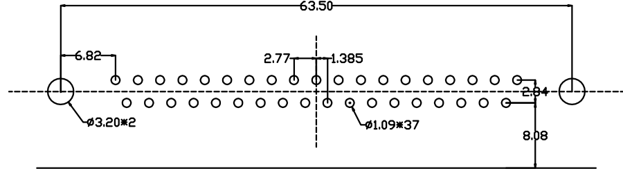
P.C.B LAYOUT
