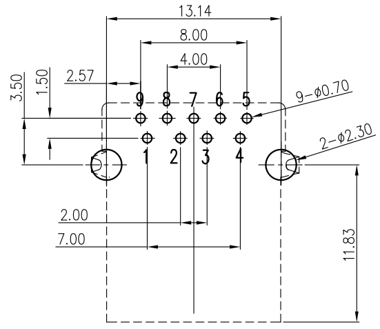
PCB LAYOUT(TOLERANCE±0.05)
